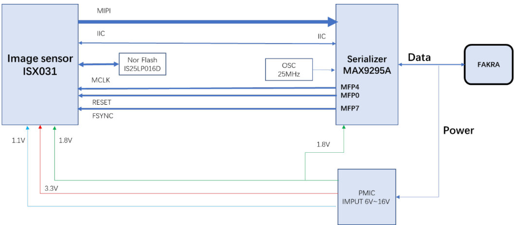
GMSL2 摄像头模组系统框图
